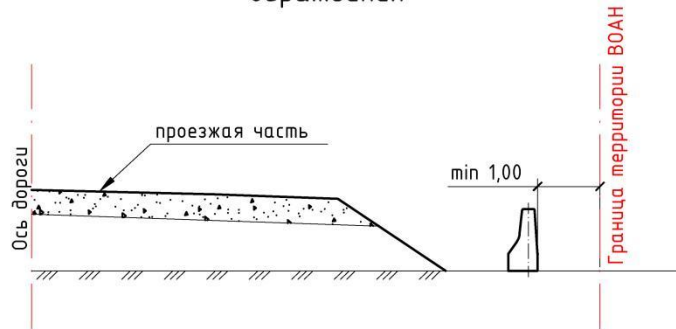
Схема установки парапетного ограждения
