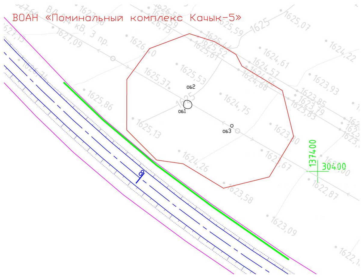
Временные ограждения ВОАН «Поминальный комплекс Качык-5»
