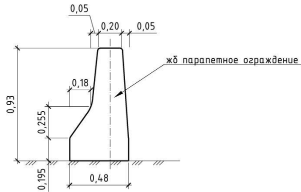
Разрез парапетного ограждения типа Нью-Джерси
